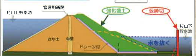
村山上貯水池堤体強化イメージ図
